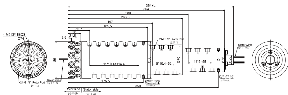
MK241S-S12(S18,S24,S36) 尺寸图 24进24出G1/8"牙+12~36路信号(2A)
