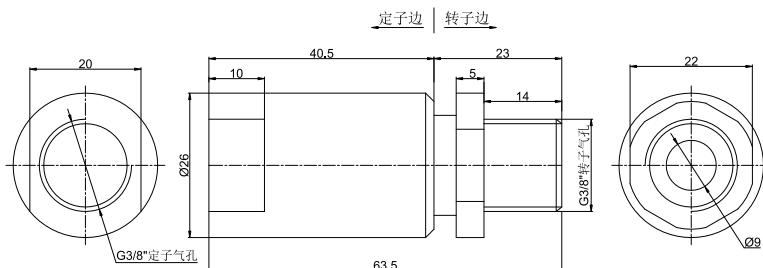
MK13A 尺寸图
