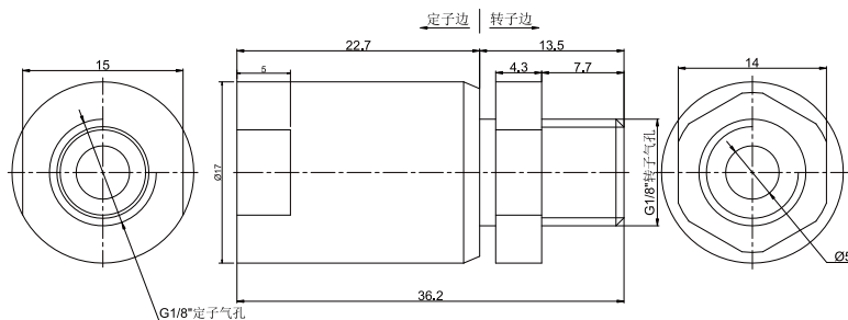
MK11A 尺寸图
