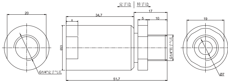
MK12A 尺寸图
