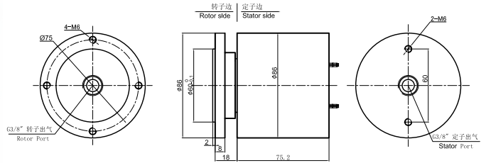
MQ100-05 尺寸图
