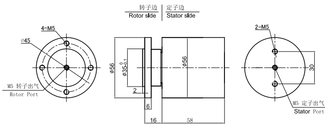
MQ100-02 尺寸图
