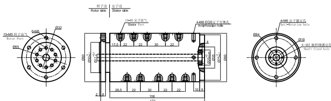
MQ1000-01 尺寸图
