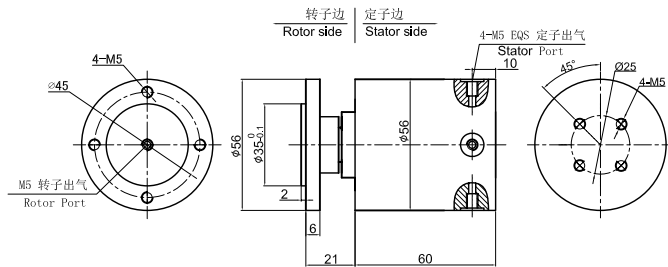
MQ104-02 尺寸图
