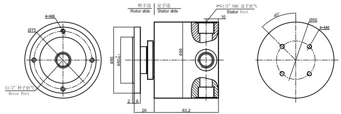
MQ104-05 尺寸图
