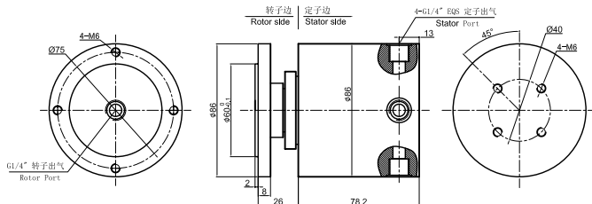
MQ104-03 尺寸图
