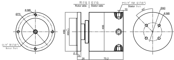
MQ104-02 尺寸图
