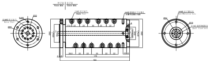
MQ1200-01 尺寸图
