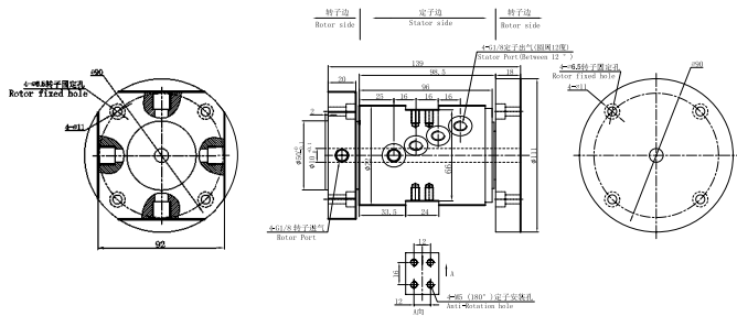
MQ400W-03 尺寸图
