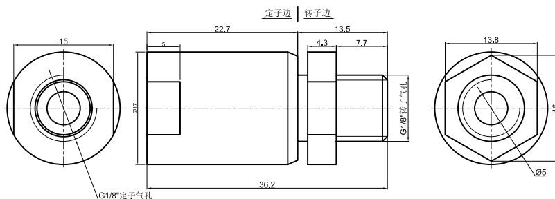
MK11A 尺寸图
