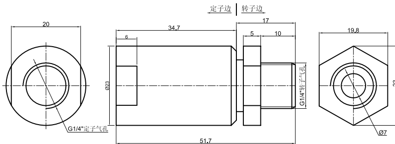
MK12A 尺寸图
