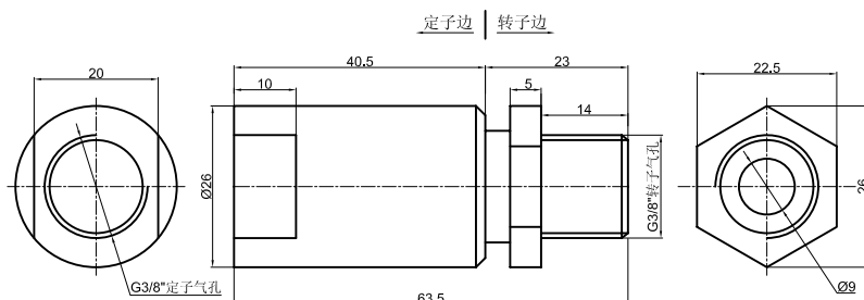
MK13A 尺寸图
