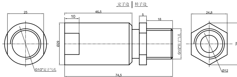
MK14A 尺寸图
